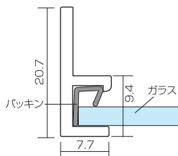
横フレーム形状
