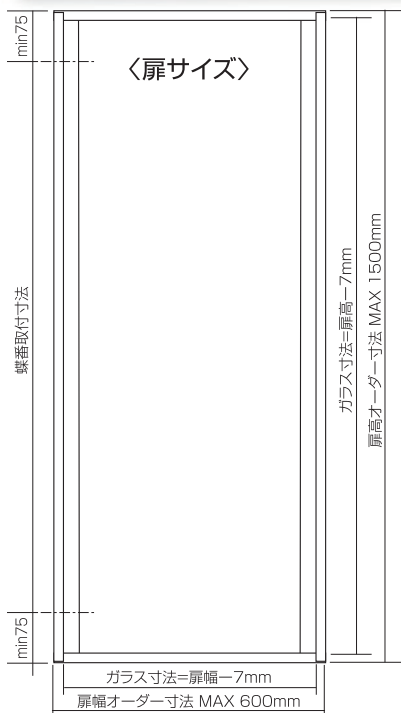
縦フレーム形状
