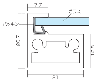
横フレーム形状
