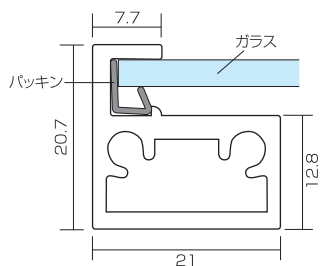
縦・横フレーム形状
